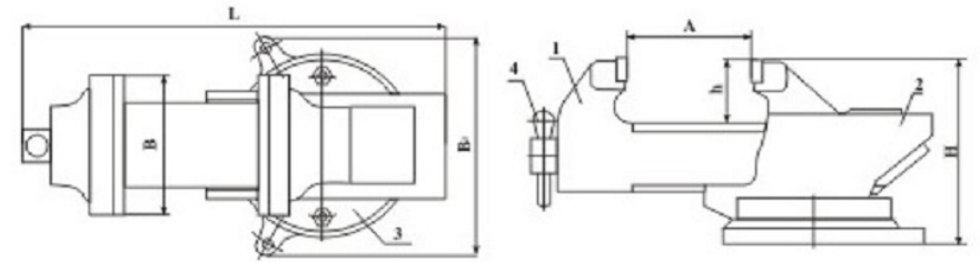
1 — губка подвижная; 2 — корпус; 3 — плита поворотная; 4 — рукоятка
